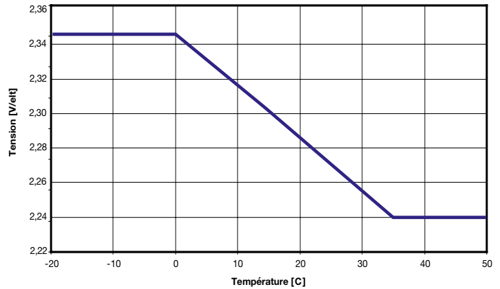
Figure 5: Sprinter PP; tension de charge en fonction de la température
