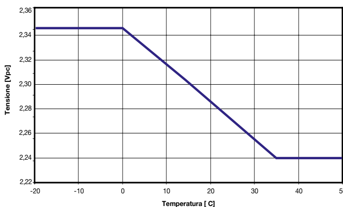
Fig. 5: Sprinter PP; tensione di carica vs. temperatura
