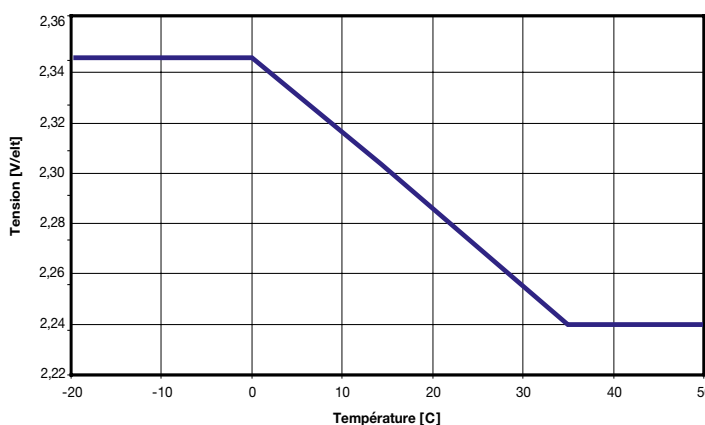
Fig. 5: Sprinter PP; tensión de carga vs. temperatura
