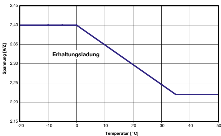
Bild 2: Marathon M-FT/PC, Sprinter P/XP/FT; Ladespannung über der Temperatur
