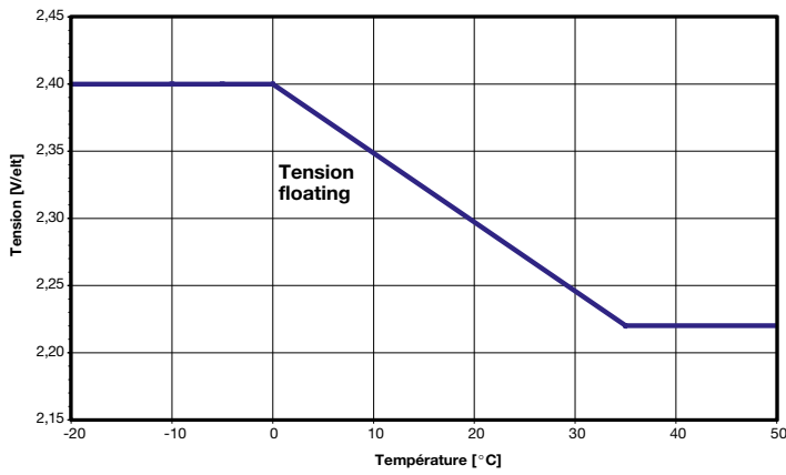
Figure 2: Marathon M-FT/PC, Sprinter P/XP/FT; tension de charge en fonction de la température
