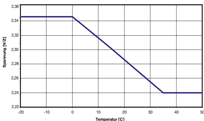
Bild 5: Sprinter PP; Ladespannung über der Temperatur
