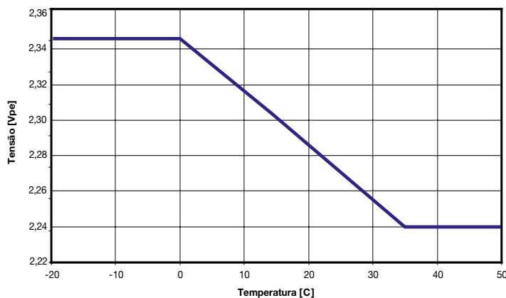
Fig. 5: Sprinter PP; tensão de carga vs. temperatura
