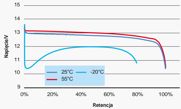
12V50Ah Rozładowanie w różnych temperaturach
