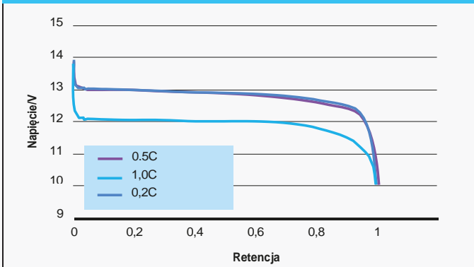
12V50Ah Krzywe rozładowania przy różnych C @RT
