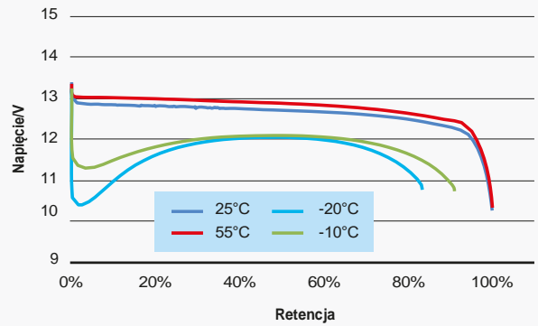
12V96Ah Rozładowanie w różnych temperaturach
